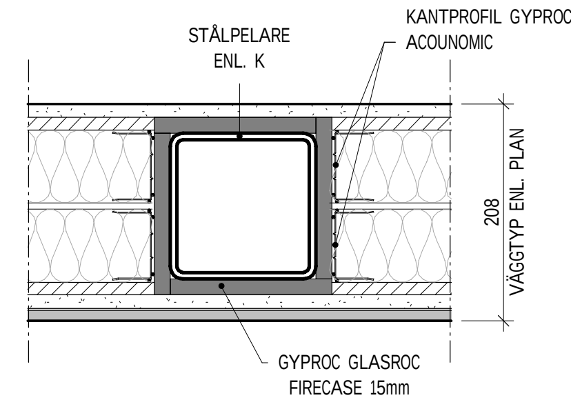
IK3 - STÅLPELARE I DUBBELREGLVÄGG 1 : 5
