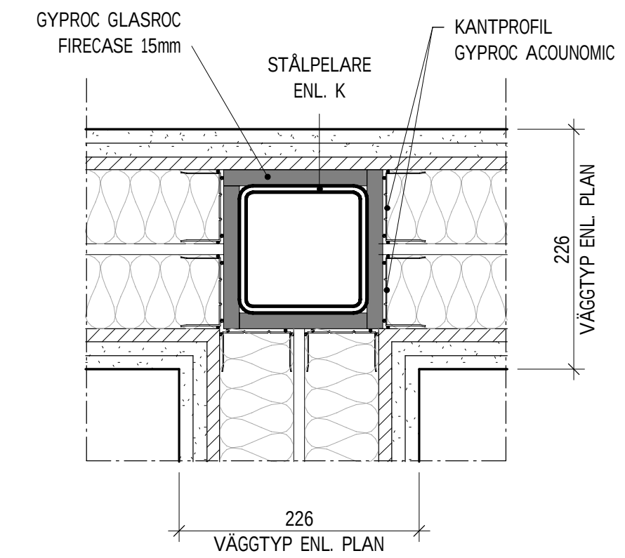
IK4 - STÅLPELARE I VÄGGKORSNING 1 : 5
