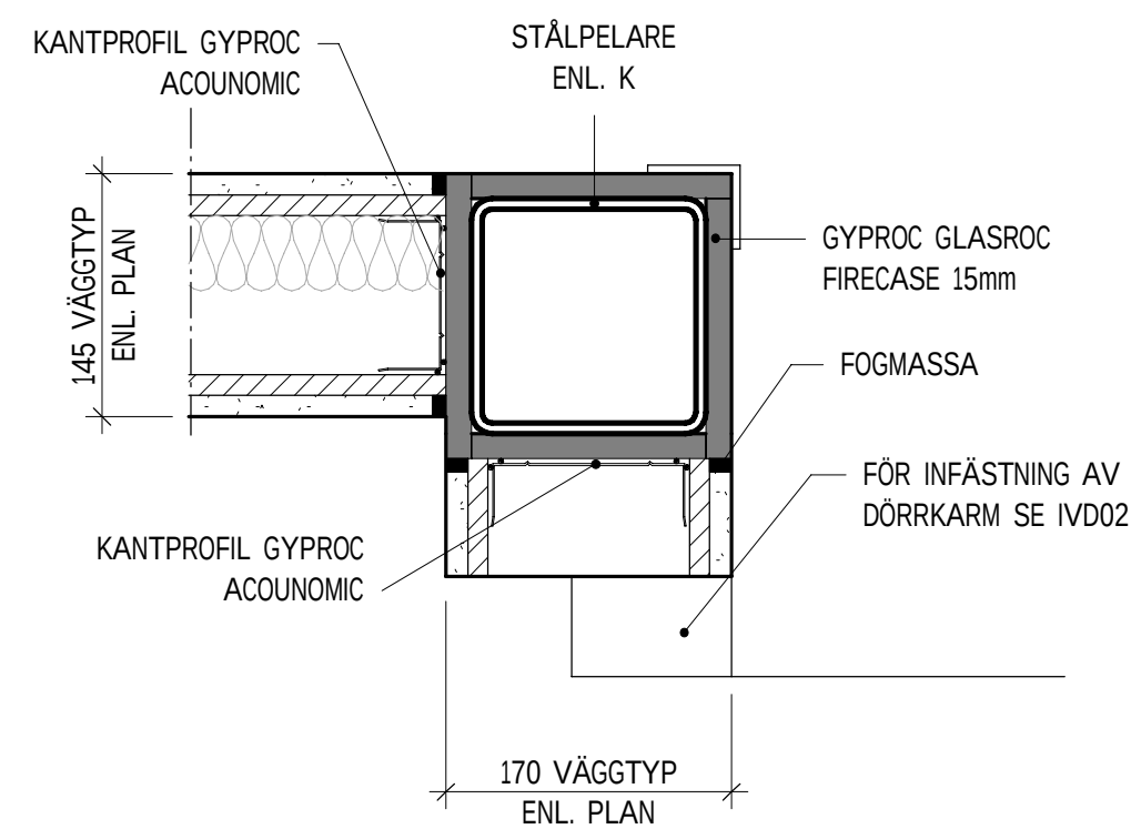
IK5 - STÅLPELARE I INNERVÄGGSHÖRN 1 : 5
