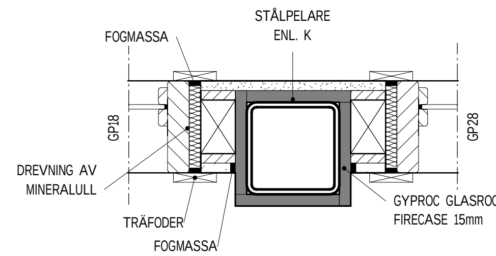
IK1 - STÅLPELARE MELLAN GLASPARTIER 1 : 5
