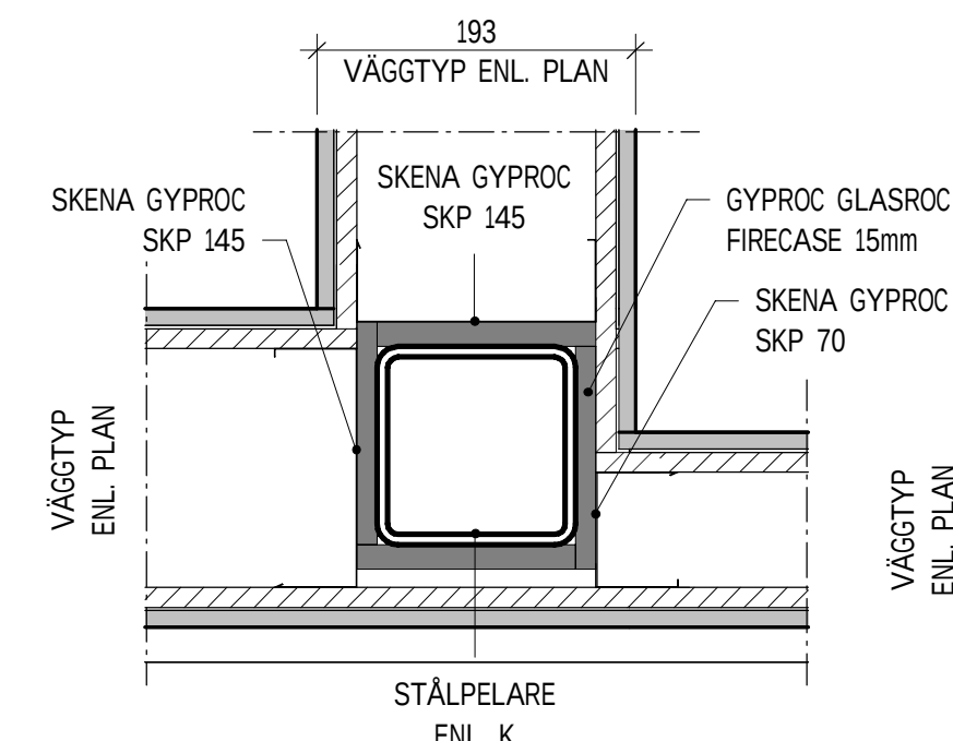
IK7 - STÅLPELARE I VÄGGKORSNING KÖK 1 : 5
