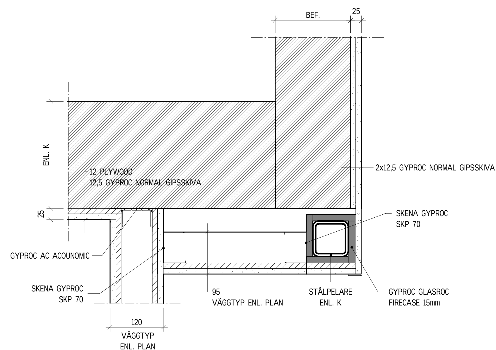
IK9 - STÅLPELARE VID BEFINTLIG VÄGG 1 : 5
