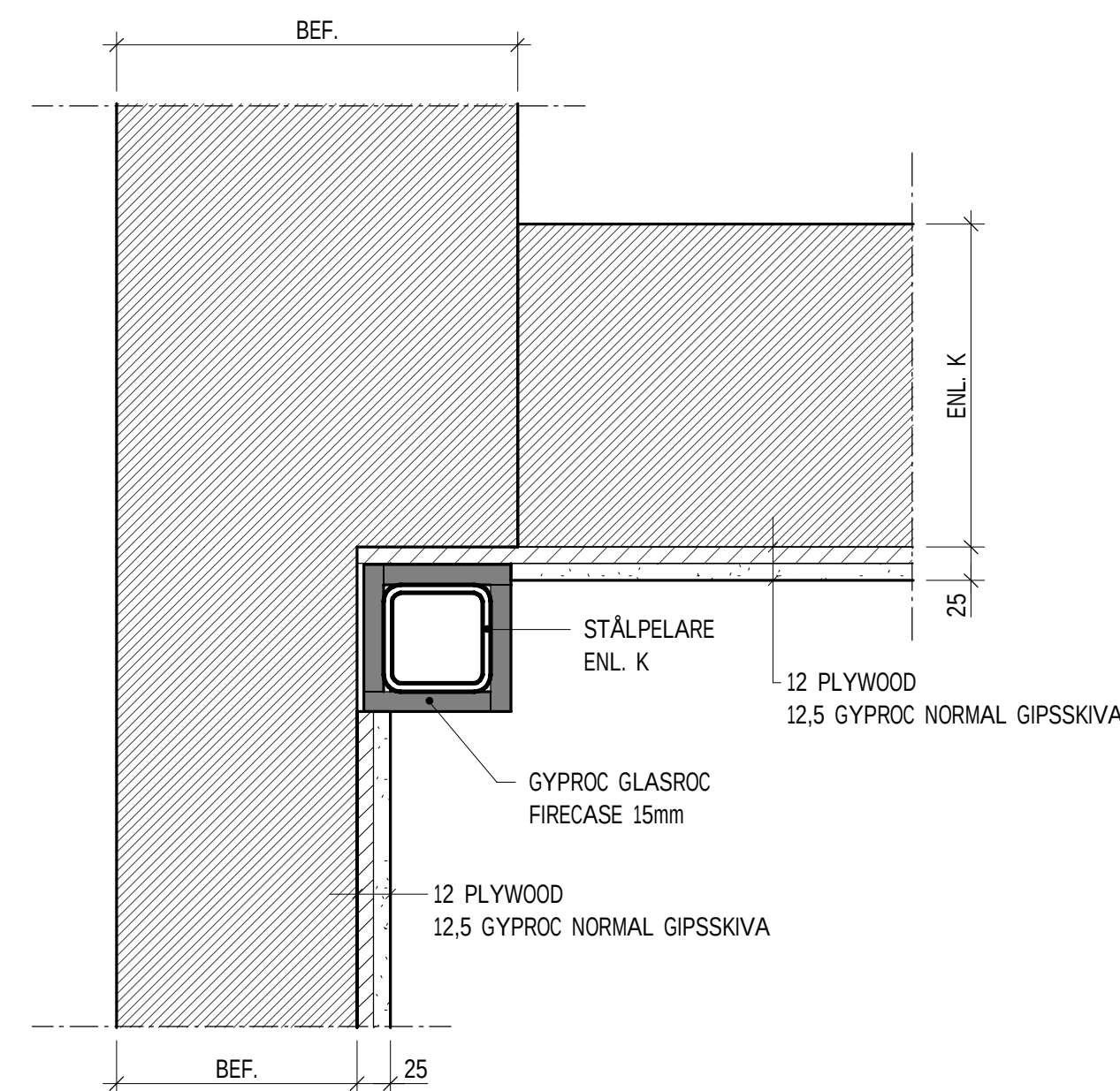
IK10 - STÅLPELARE VID BEF. VÄGGHÖRN 1 : 5
