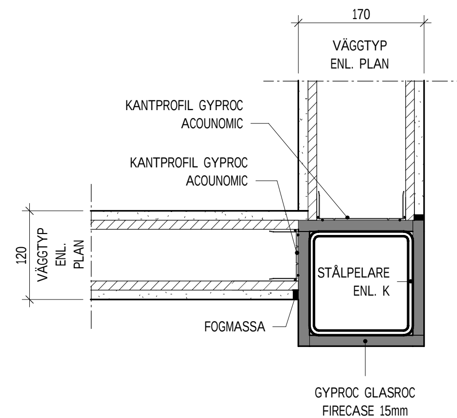
IK6 - HALVT UTSTICKANDE PELARE 1:5
