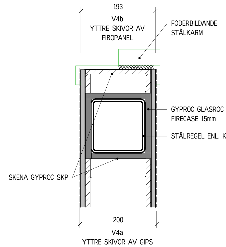
IK2 - STÅLPELARE I INNERVÄGG 1:5
